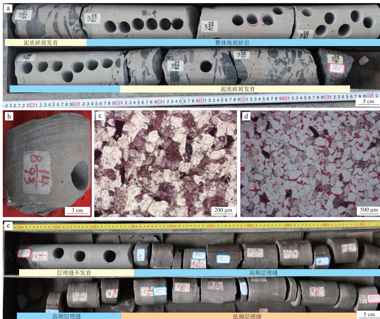
图5 四川盆地川西坳陷须二段致密碎屑岩储层沉积、成岩与破裂非均质性特征照片
